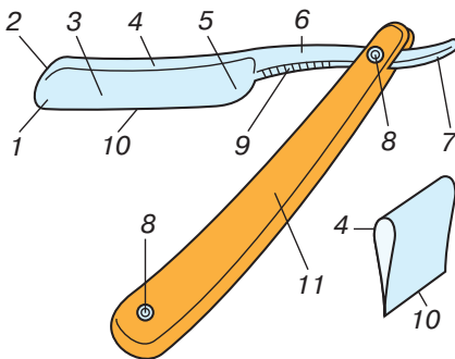
Рис. 2.16. Складові частини небезпечної бритви:
