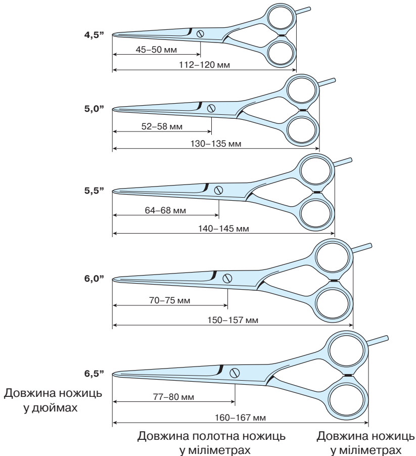
Рис. 2.10. Шаблон визначення розміру полотен перукарських ножиць
